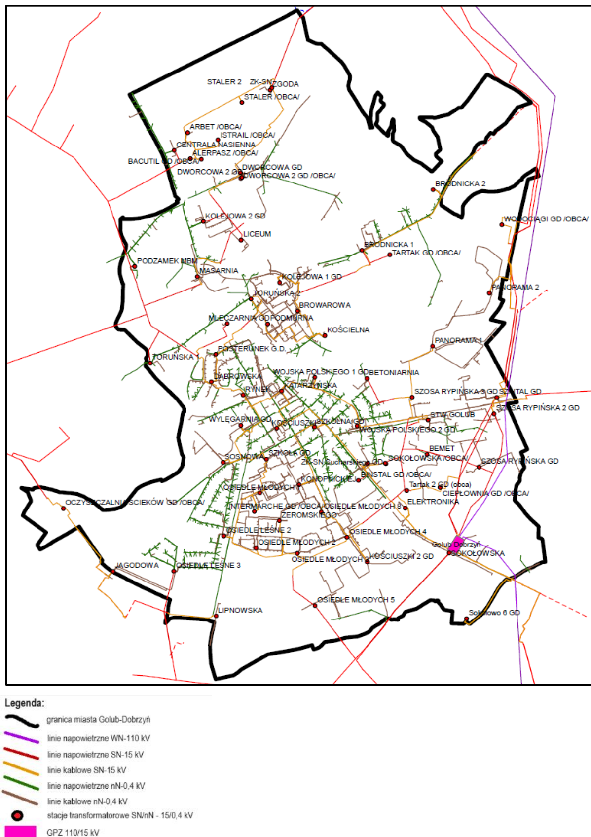
Rysunek 6. Schemat sieci energetycznej przebiegającej przez miasto Golub-Dobrzyń
